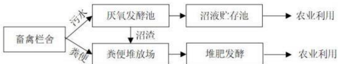
图 4-2 畜禽粪污厌氧+就近还田模式
